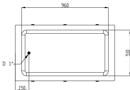
Boven aanzicht
