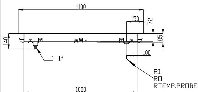
Zij aanzicht
